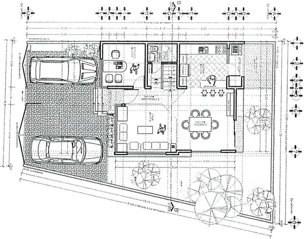
PLANTA BAJA.
