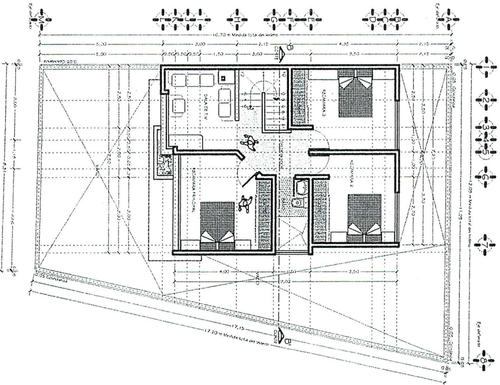
PLANTA ALTA.
