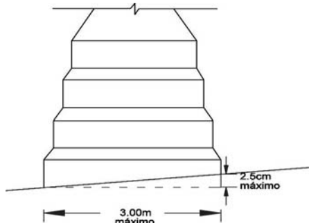
DIBUJO 4.1.3-B. ESCALÓN Y DESCANSO CON PENDIENTE - VISTA FRONTAL
